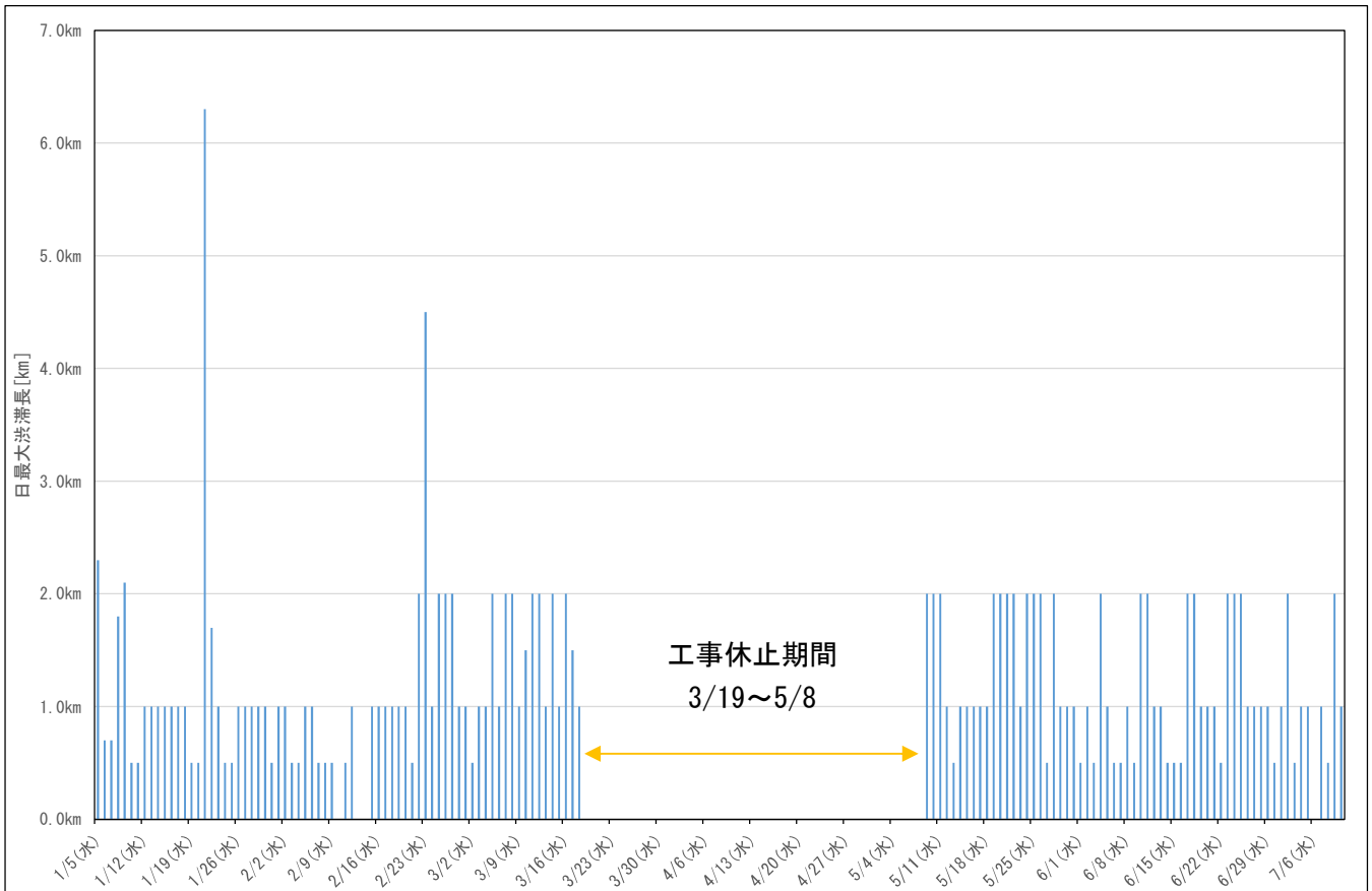
日最大渋滞長について（E84 西湘 BP 橋 IC～小田原 IC 間下り線）
